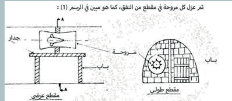
مقتطف من مذكرة تثبيت الهوائيات المسماة "هوائيات معزولة"، تم تصميمها بواسطة مكتب دراسات المنجم
